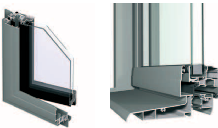
Variante CP 50-Mb - Solution monobloc pour doublage intérieur de 100, 120, 140 et 160 mm
